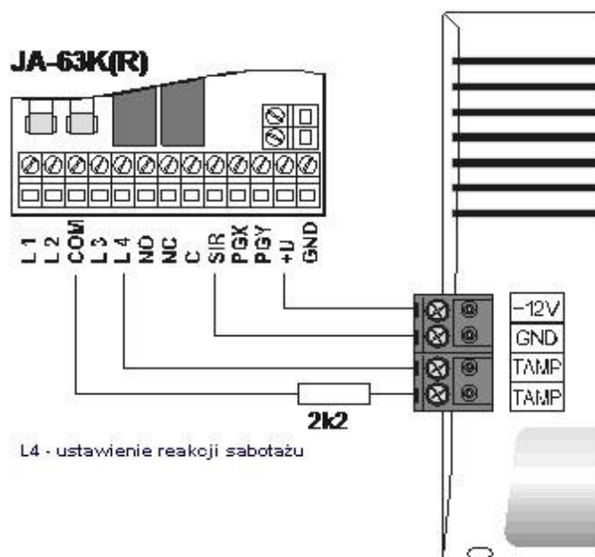
Rysunek 2. Przykład podłączenia syreny z centralą JA-63K(R)
